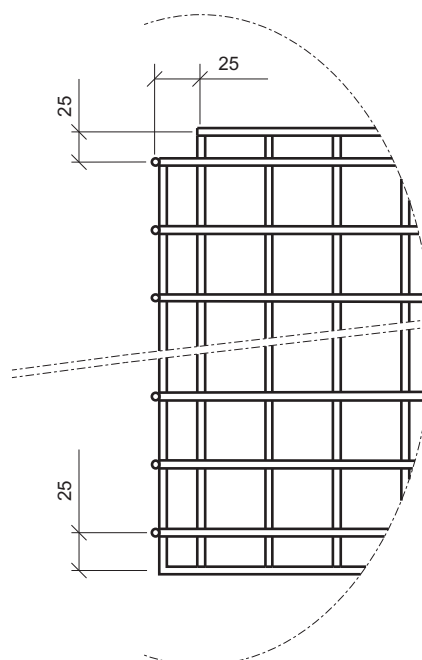
Détail D
