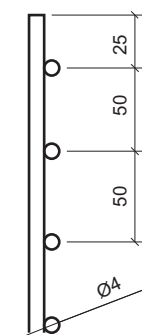
Détail B
