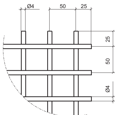
Détail C
