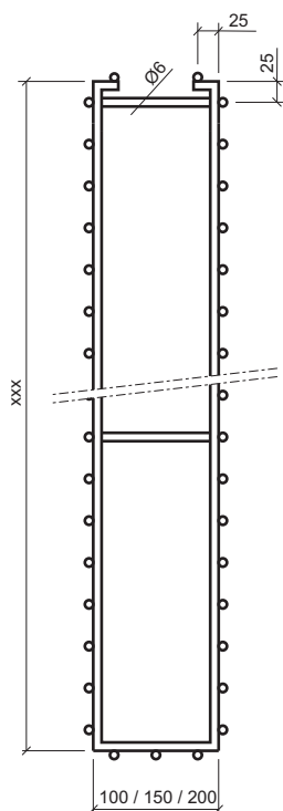
Détail C
